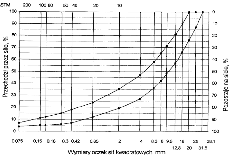
Rys. 1. Krzywe graniczne uziarnienia mieszanki mineralnej BA od 0 do 25 mm podbudowy nawierzchni drogi o obciążeniu ruchem od KR 3 do KR 6
