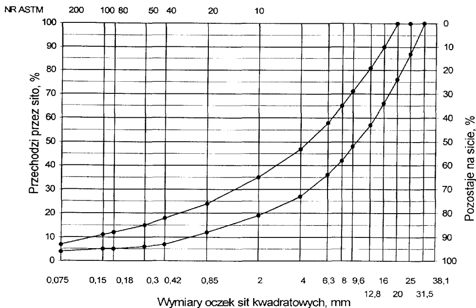
Rys. 1. Krzywe graniczne uziarnienia mieszanki mineralnej BA od 0 do 25 mm podbudowy nawierzchni drogi o obciążeniu ruchem KR 6
