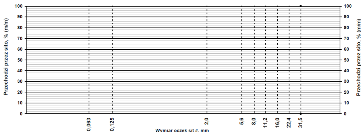
Rys. 1. Przykładowy układ współrzędnych do sporządzenia wykresu uziarnienia zaprojektowanej mieszanki mineralnej
