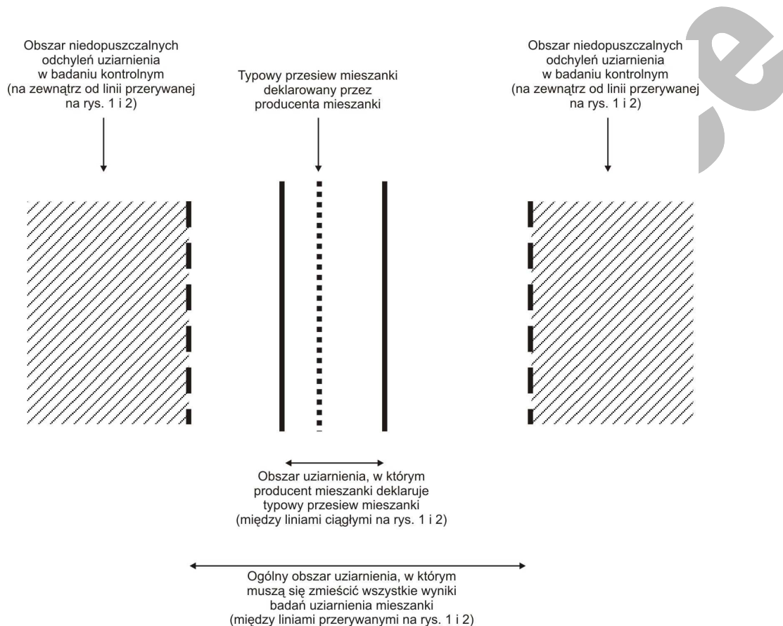
Rysunek A.1 Zastosowanie wartości deklarowanej przez dostawcę [producenta]
